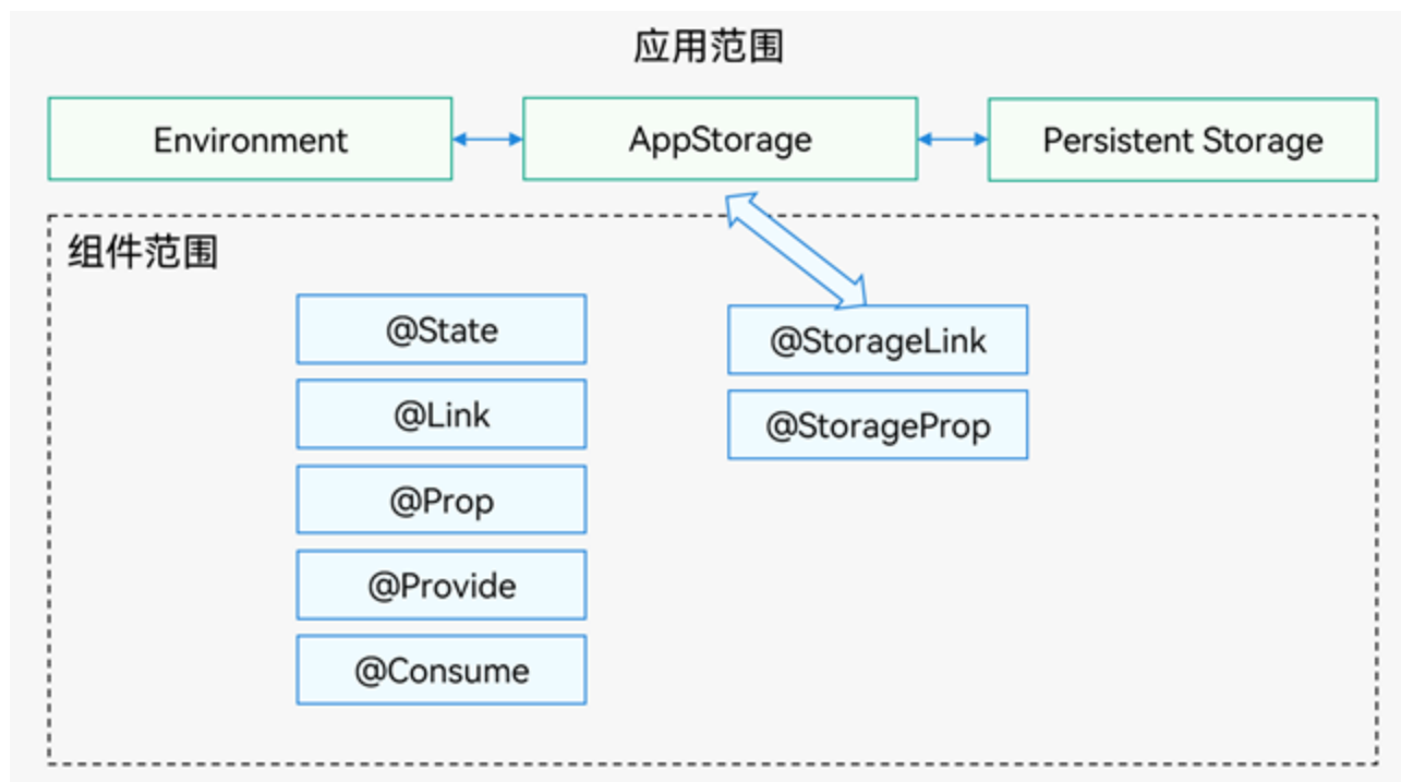
图 5-2：状态管理
