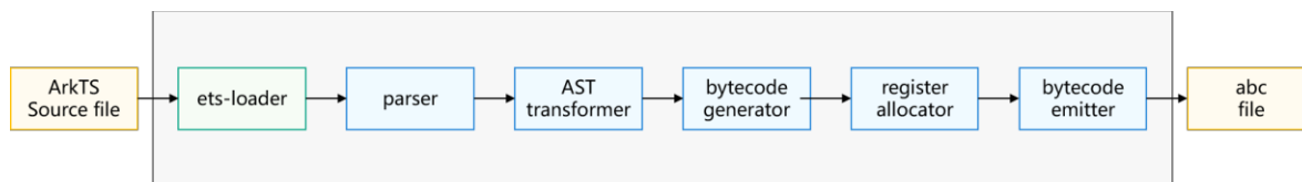
图 4-6：方舟编译器
